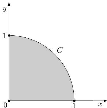
FIG. 1. Le cercle C d'équation x^2 + y^2 = 1 FIG. 2. L'hyperbole H d'équation xy = 1
